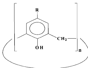
Figura 1. Structura unui compus calixarenic
