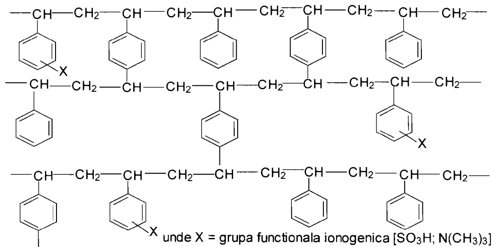
Figura 2. Structura unei rasini schimbatoare de ioni
