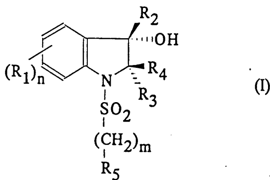
isomère cis
