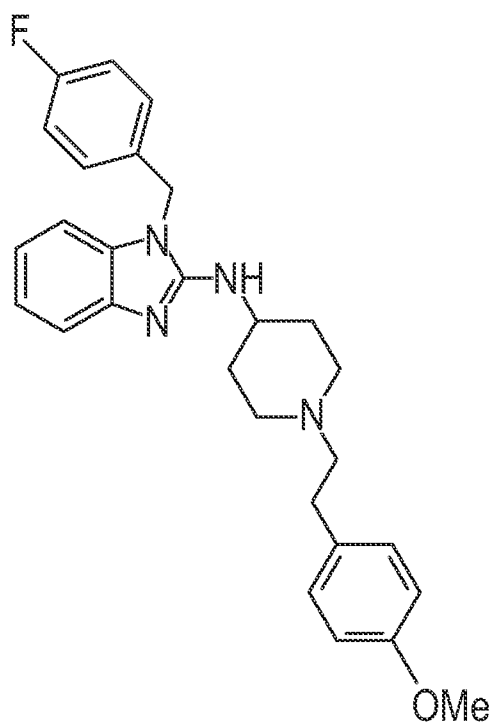
Astemizole (1)
