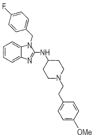
Astemizole (1)
