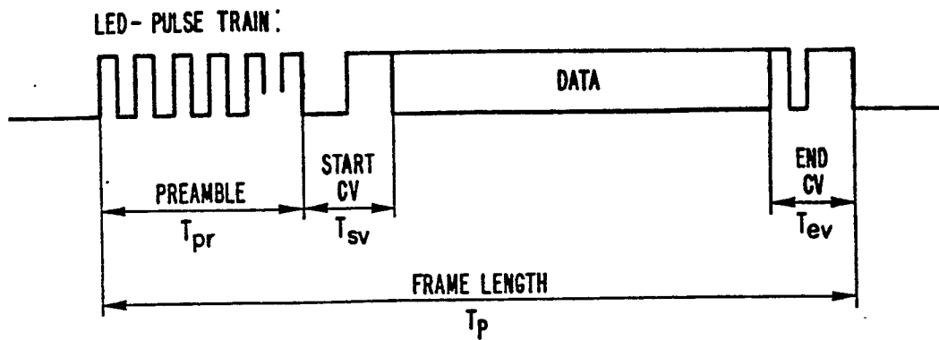
FIG. 3 FRAME FORMAT
